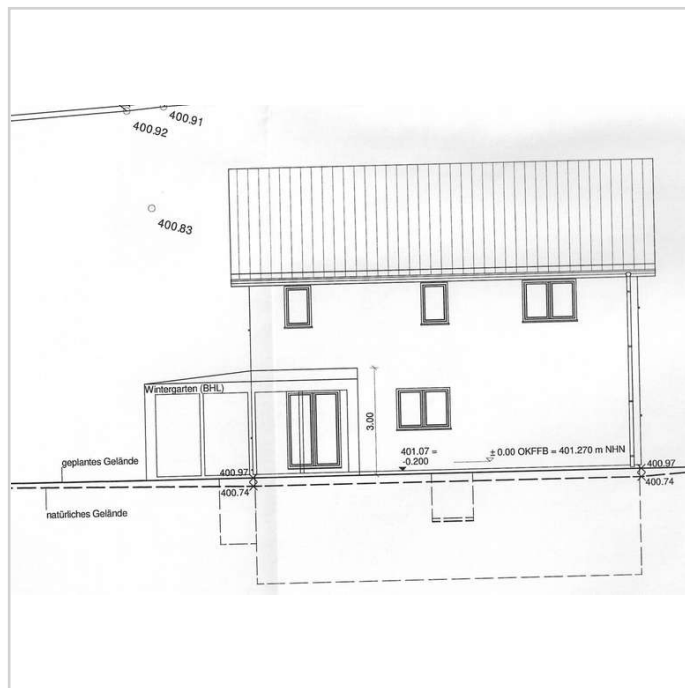
Süd
