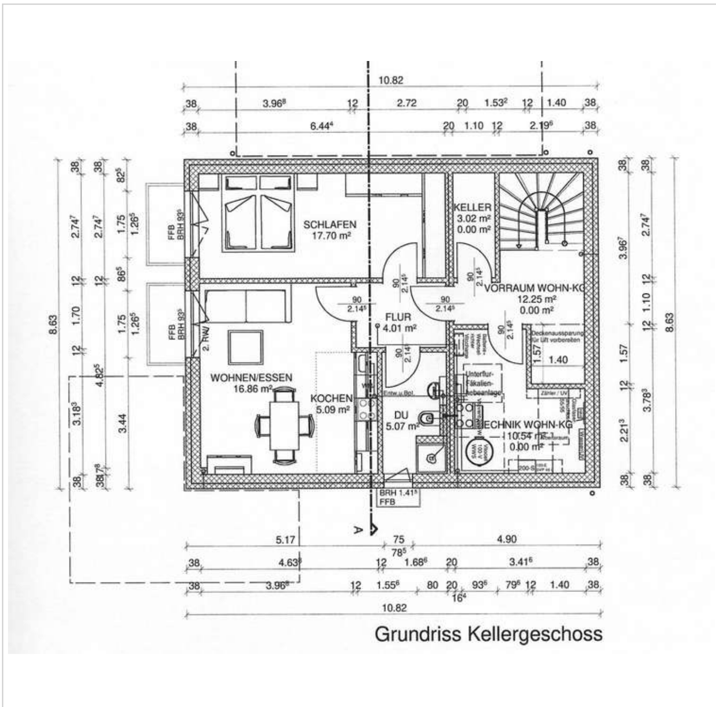
Grundriss KG
