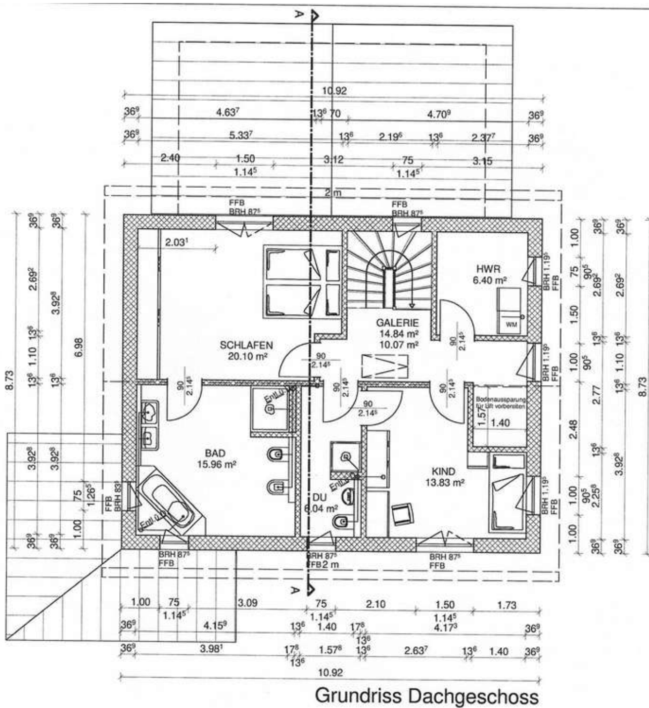
Grundriss DG
