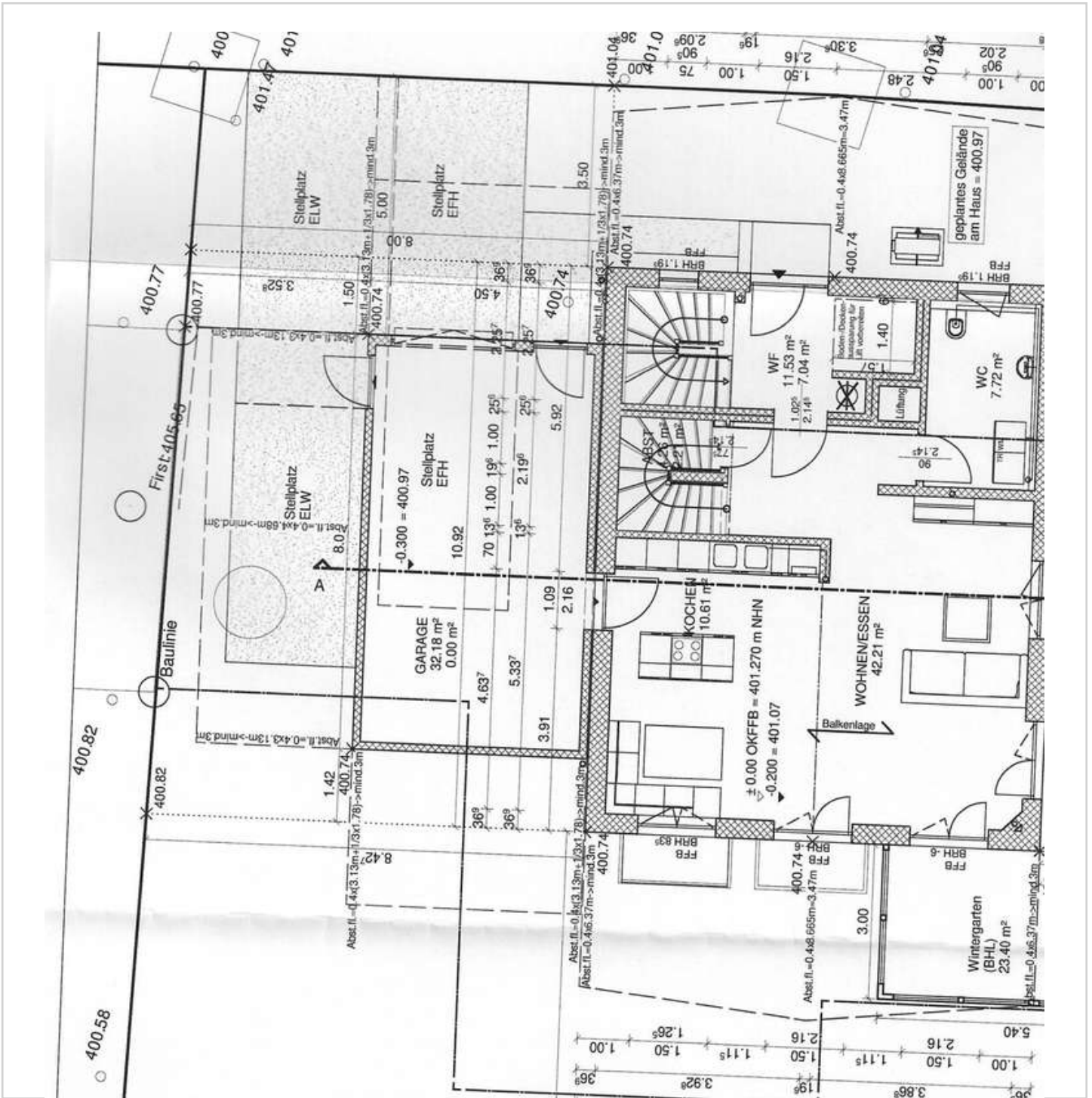
Grundriss EG
