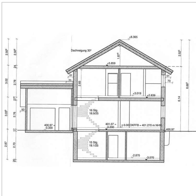
Nord Ansicht
